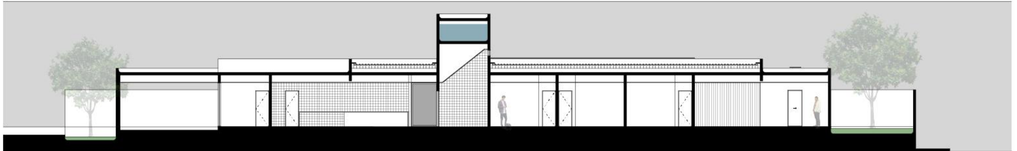
CORTE AA
