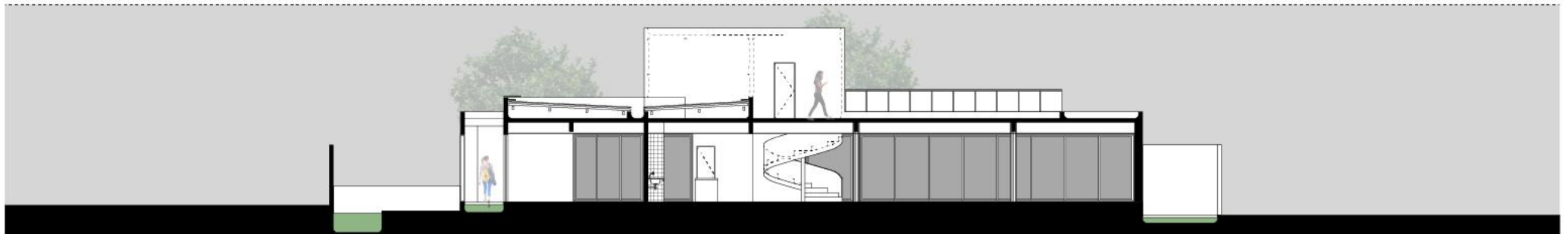
CORTE BB
