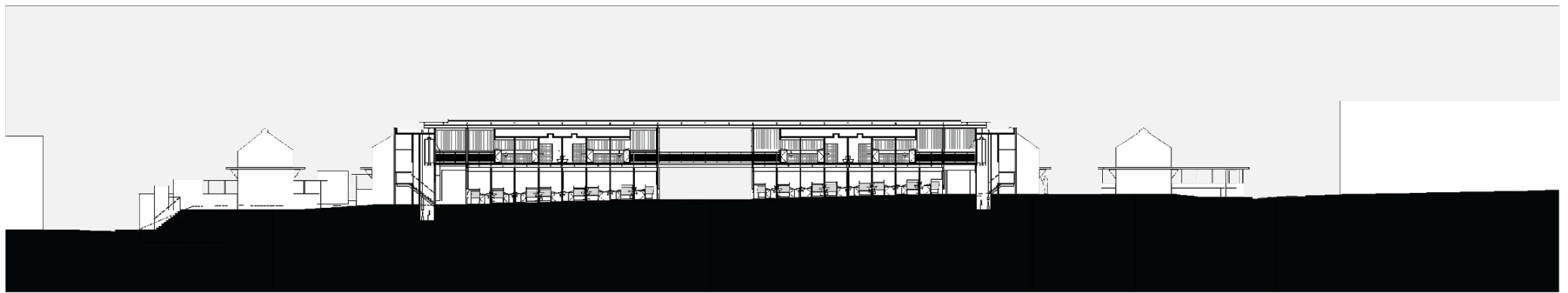
CORTE AA
